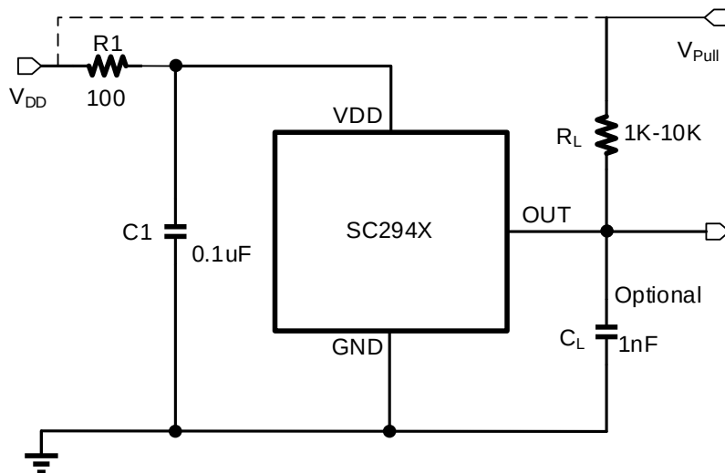
图 6 典型应用线路图
