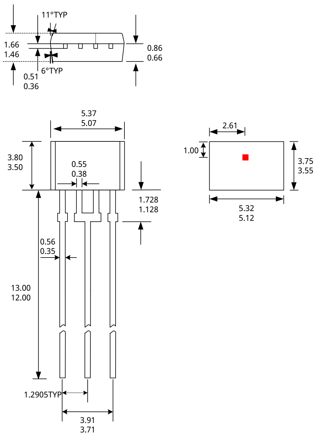
VB-S PKG
