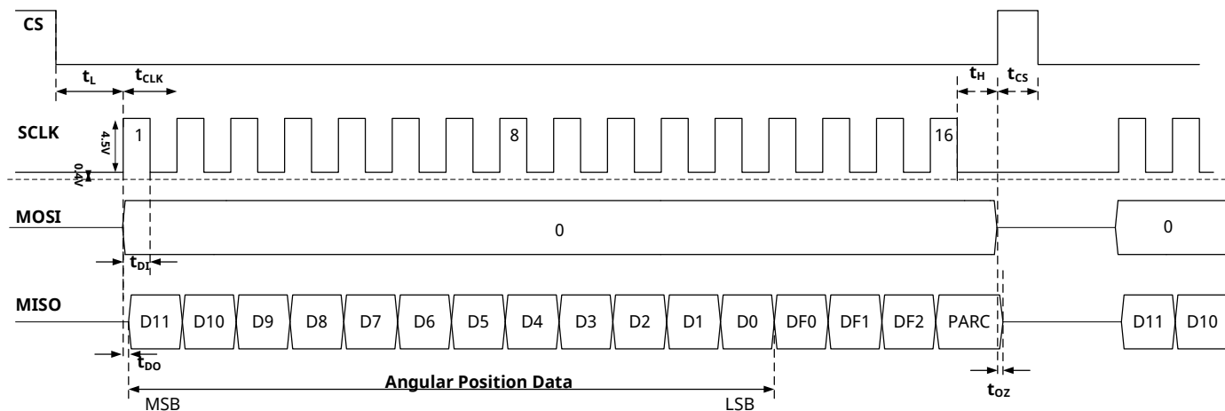
图 7: SPI 时序图
