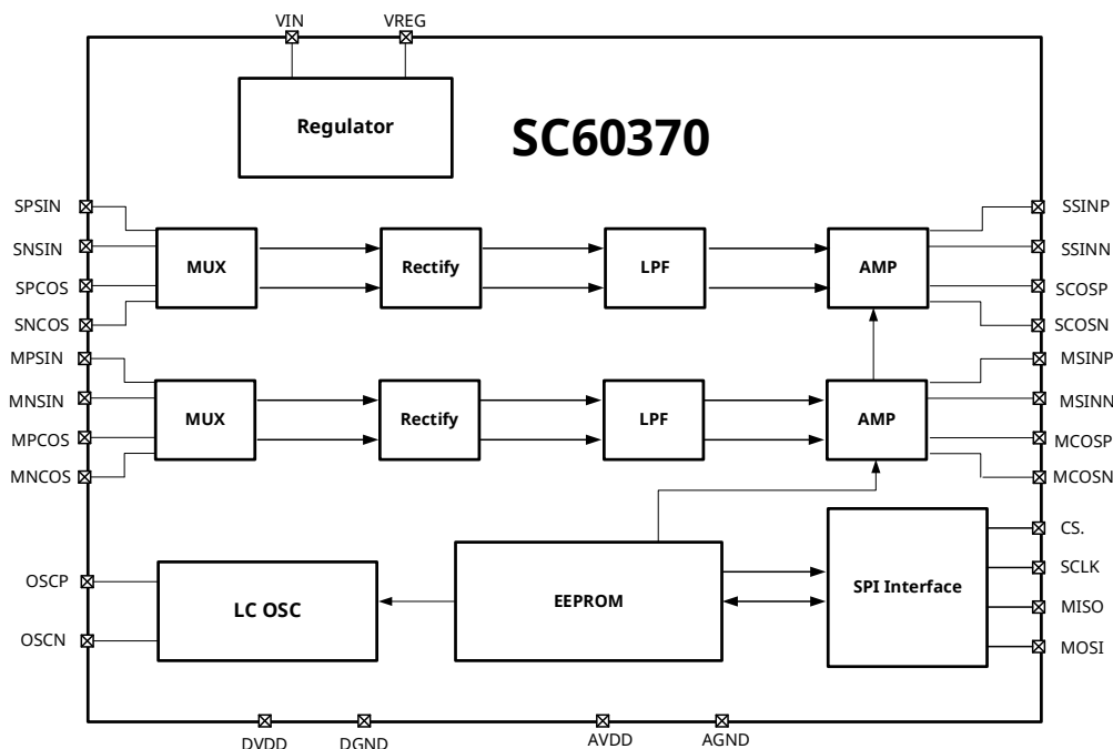
图 3：功能框图
