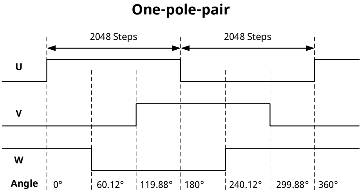
图 6: 1 对极 UVW 波形图
