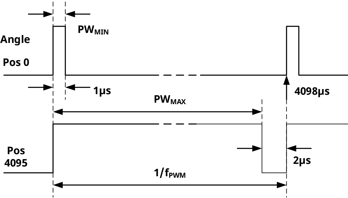
图 8：PWM 波形图
