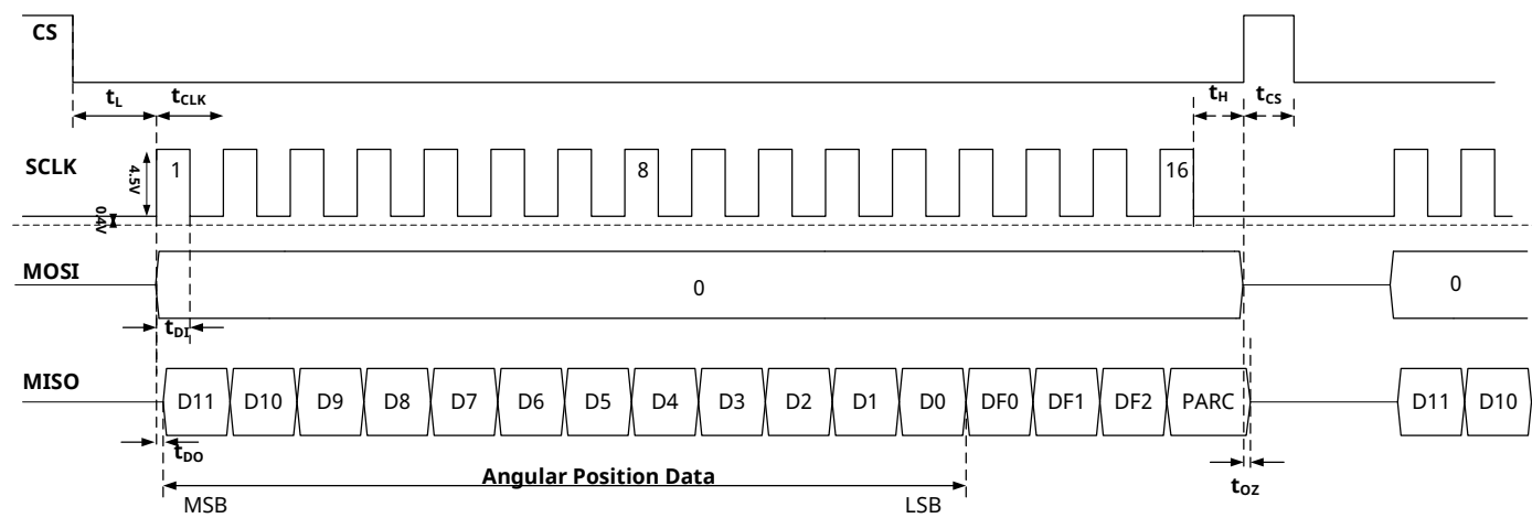
图 7：SPI 时序图
