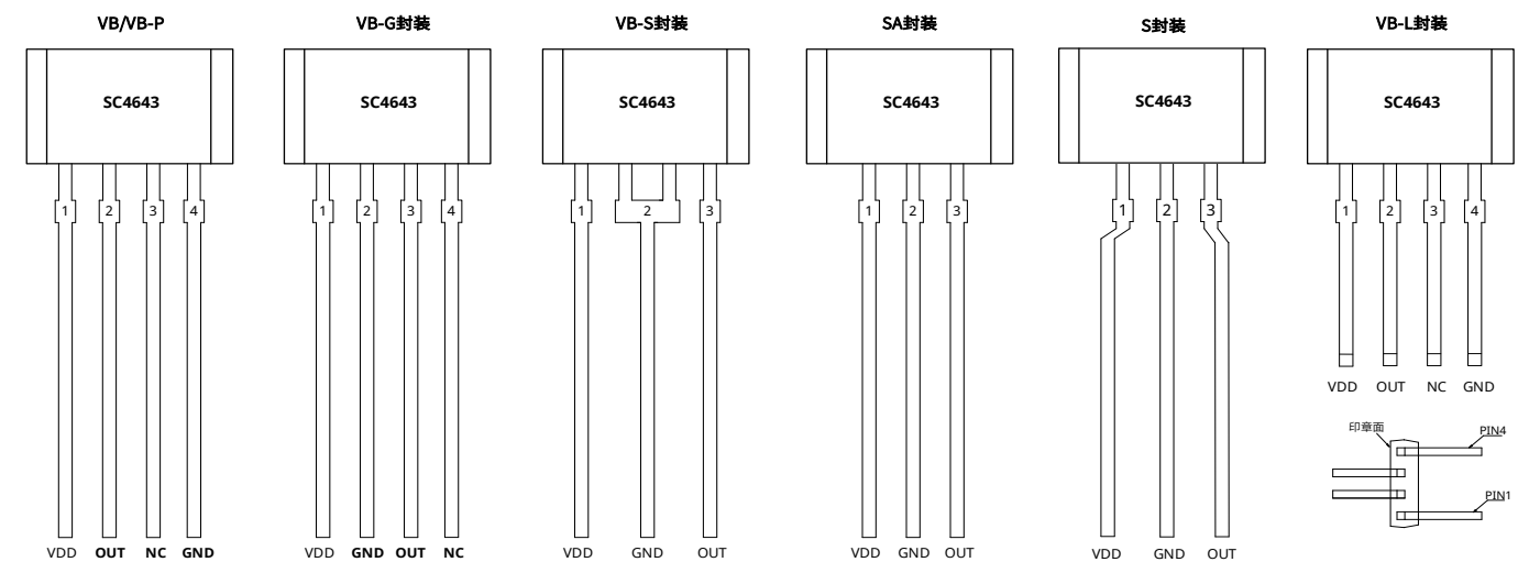
图 2. 封装俯视图
