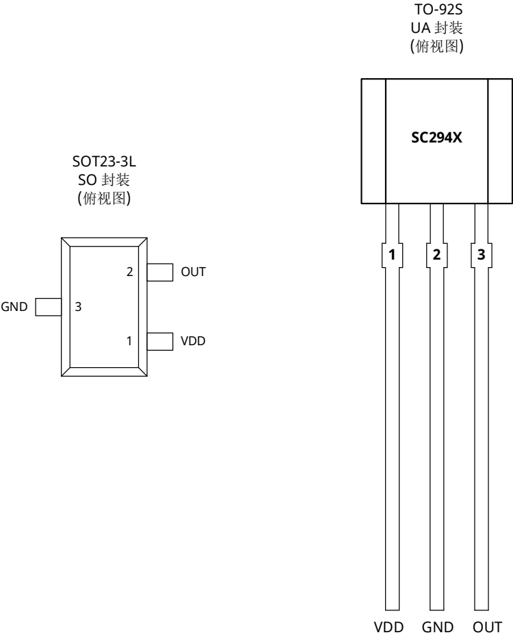
图 2: 引脚定义图
