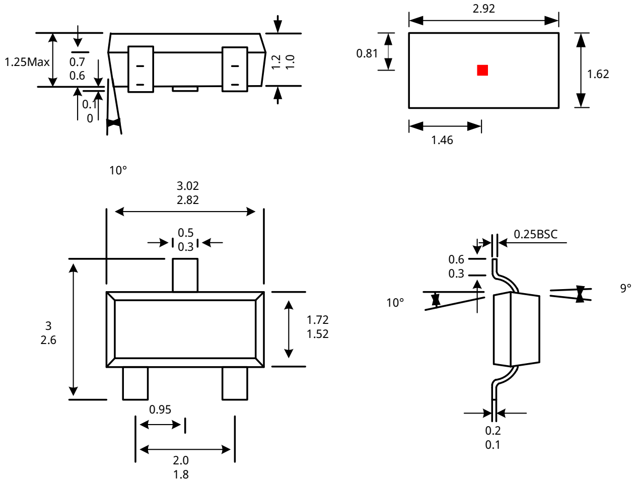
3-脚 SOT23-3L 封装
