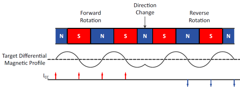
图 18 方向改变
