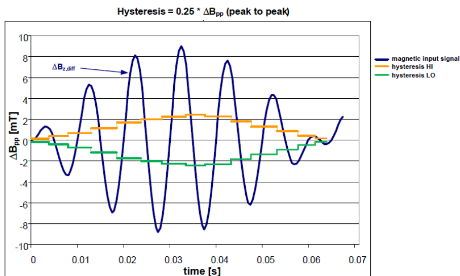
图 17 自适应迟滞
