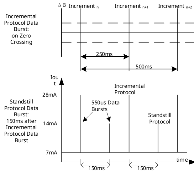
图7 静止协议
