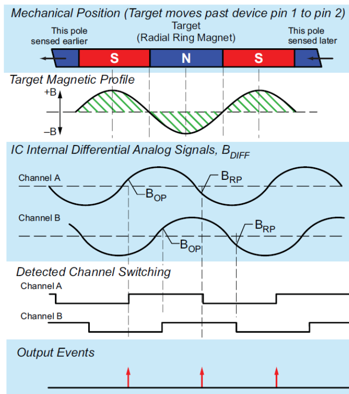
图 16 方向检测
