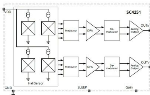
SC4251 框图
