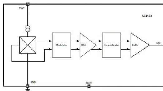
SC410X 框图
