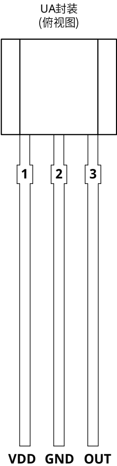
图 2 引脚描述
