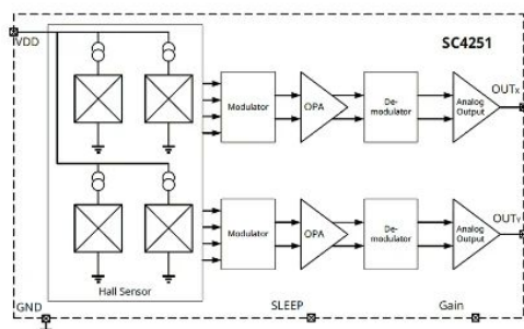
SC4251 框图
