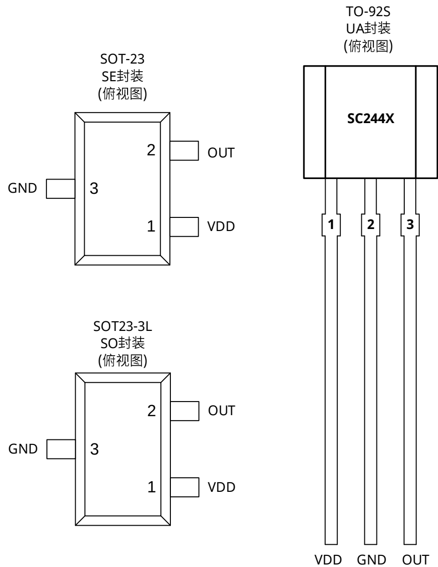
图 2：引脚定义图
