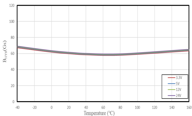
SC2443 B_{HYS} VS. Temperature
