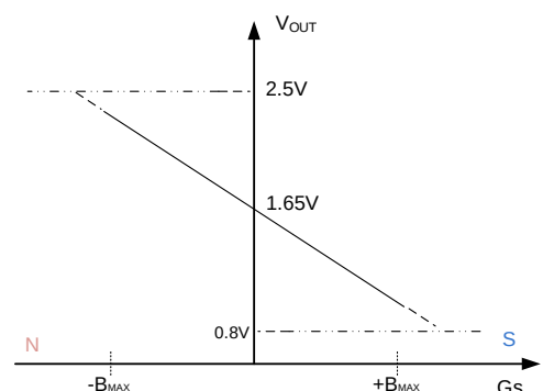
Fig 5-4. SOT23-3L PKG Output-3.3V
