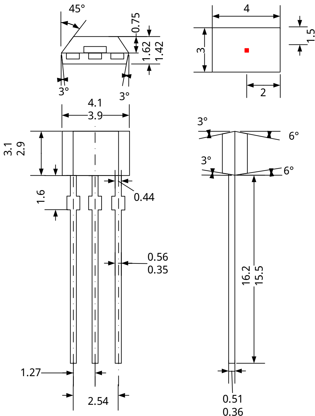
UA 封装
