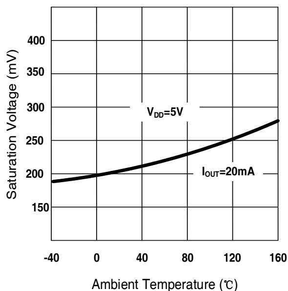
V_{Q(sat)} vs T_A
