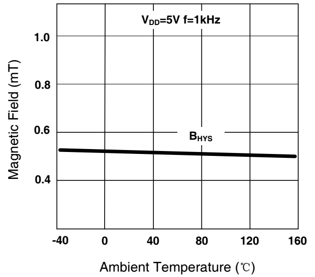
SC2430 B_{HYS} vs T_A
