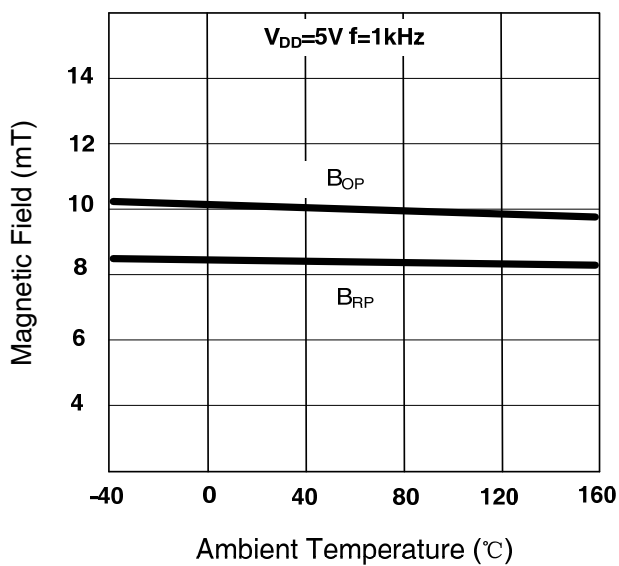
SC2436 B OP and B RP vs T A
