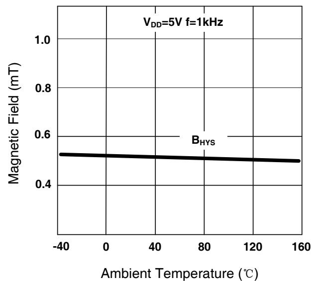
SC2432 B_{HYS} vs T_A
