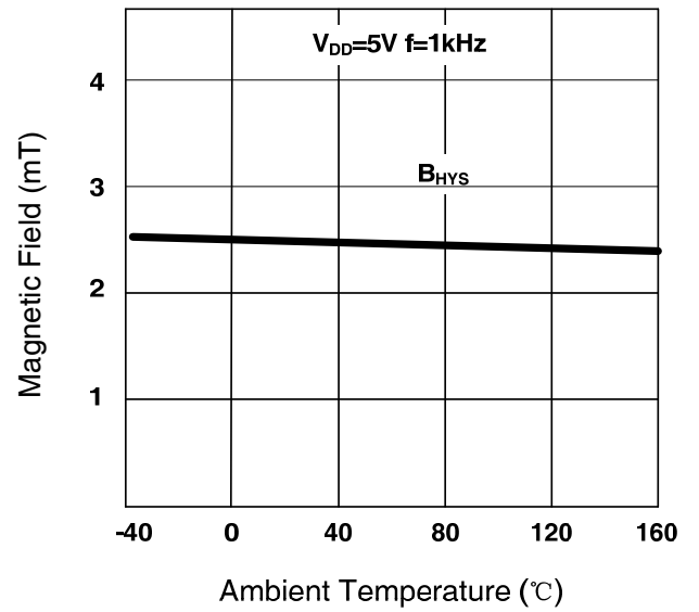
SC2438 B_{HYS} vs T_A
