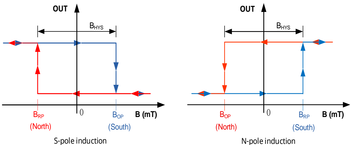
图 5 传输曲线图
