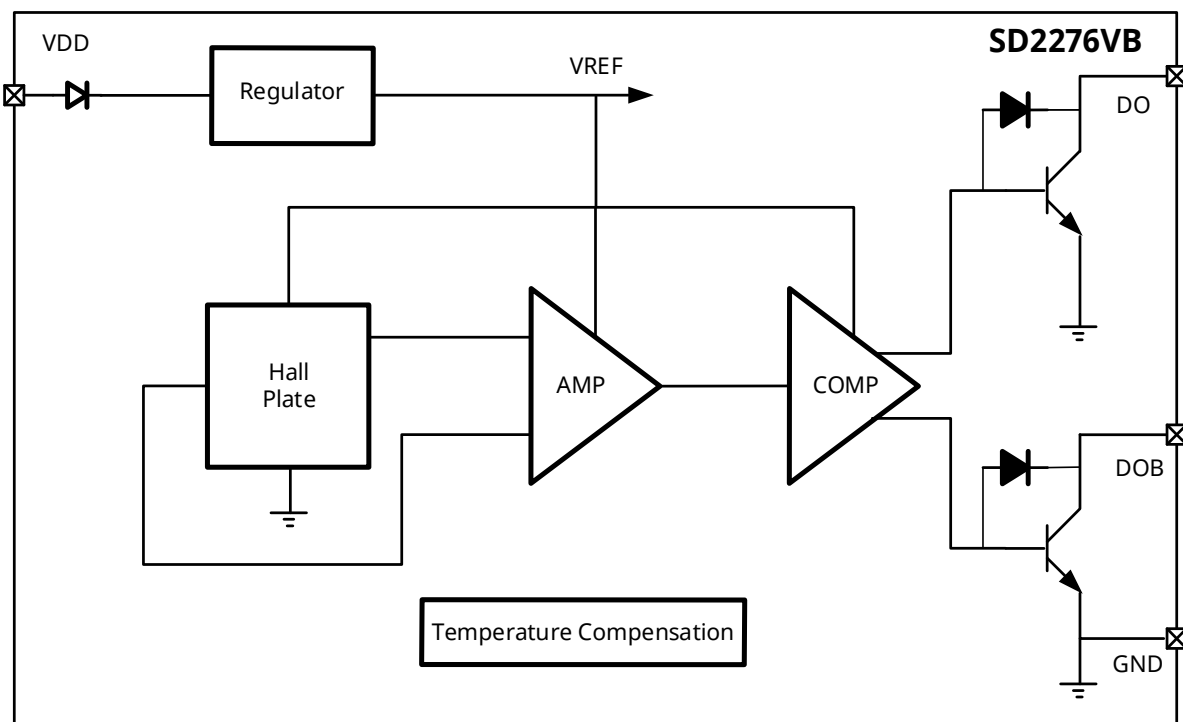
图 3: 功能框图
