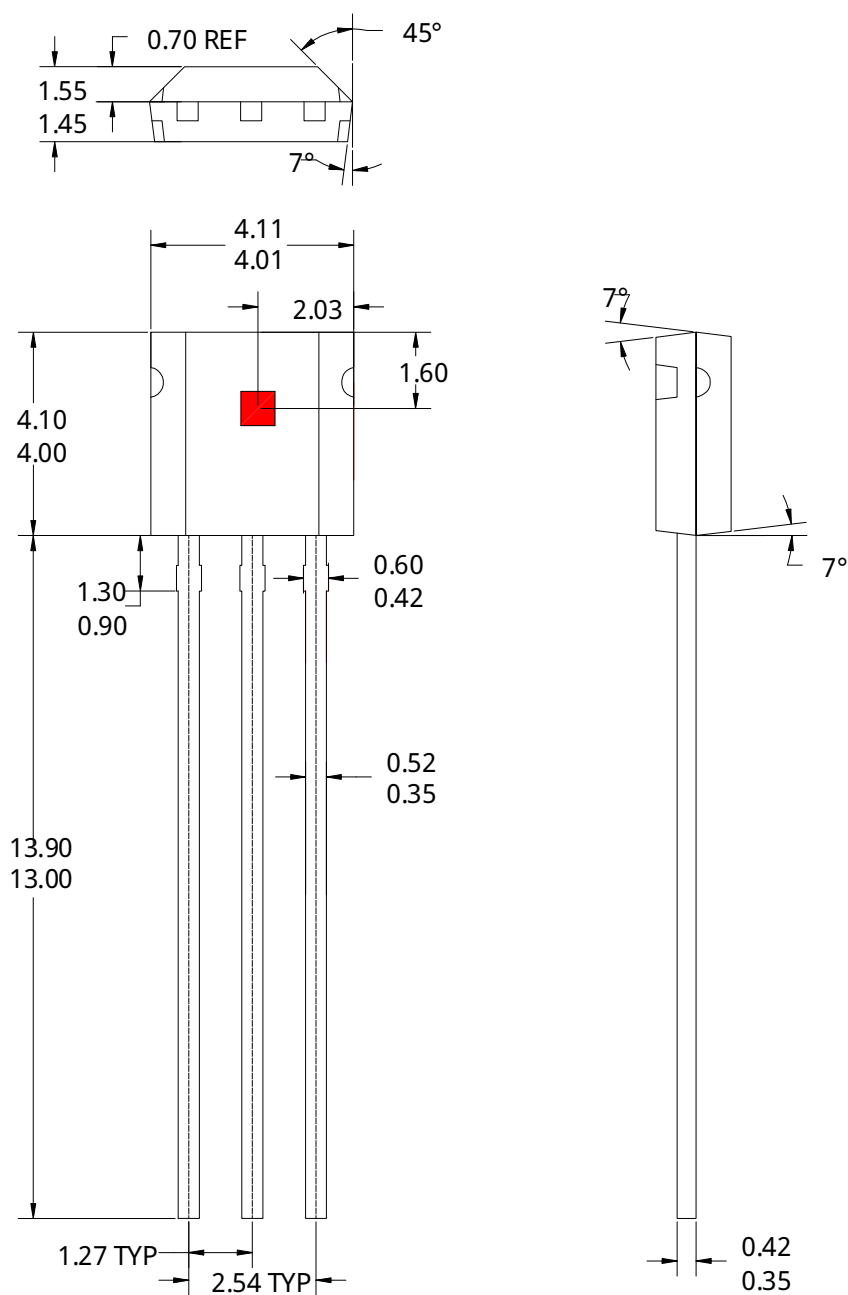
图 6: 封装尺寸图 (单位: 毫米)
