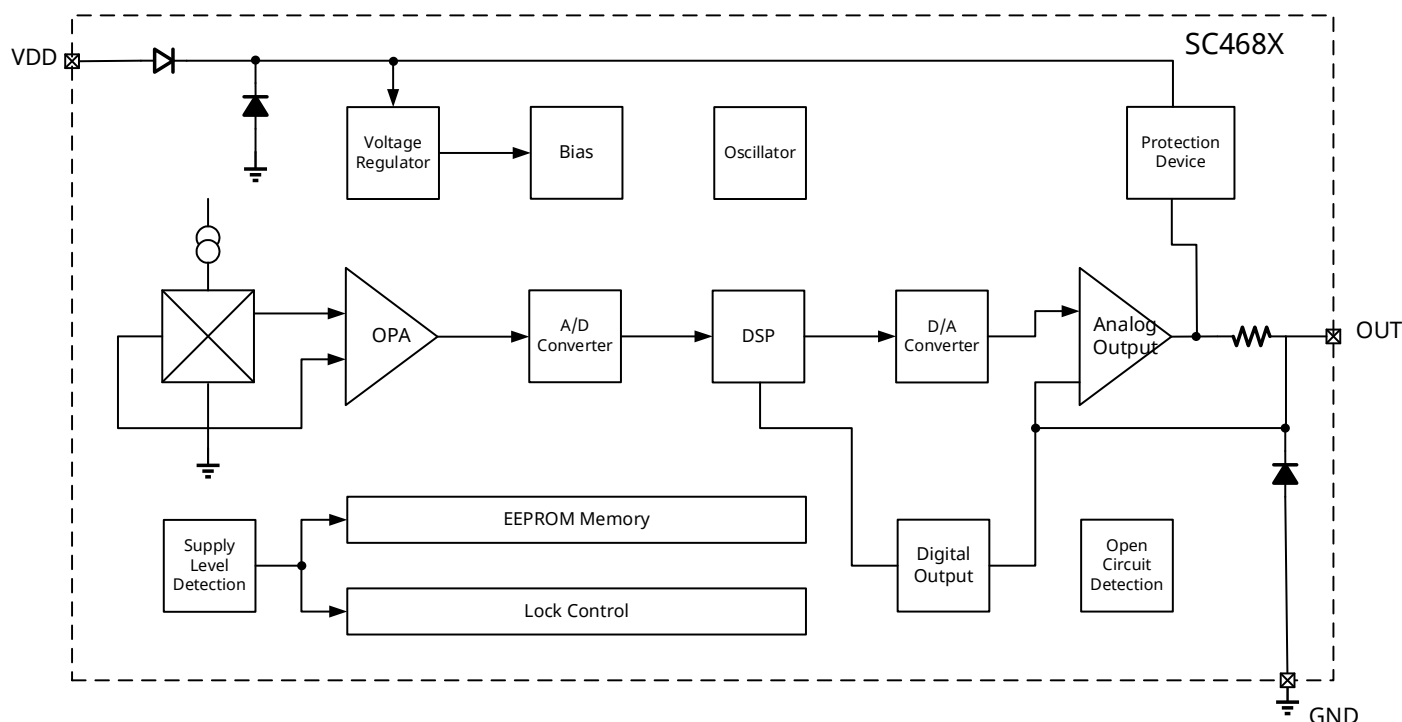
图 3：功能框图
