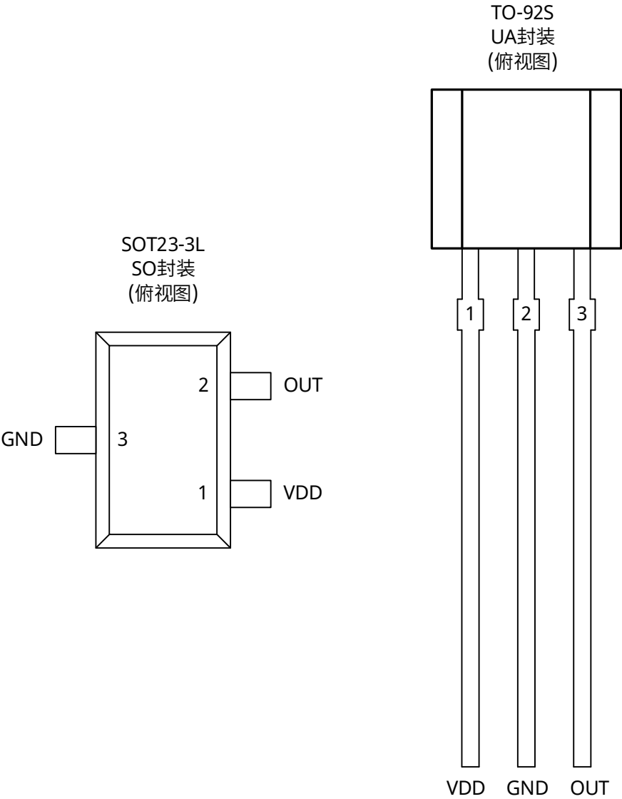
图 2 引脚描述
