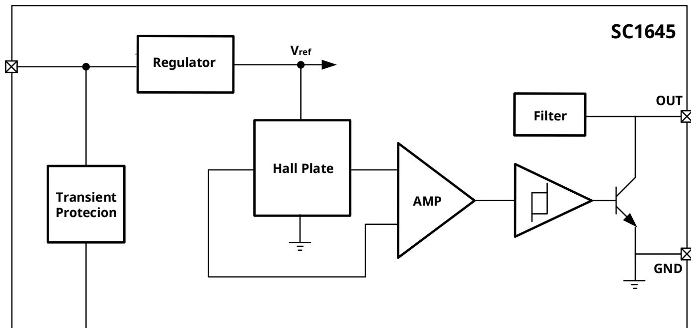
图 3 功能框图
