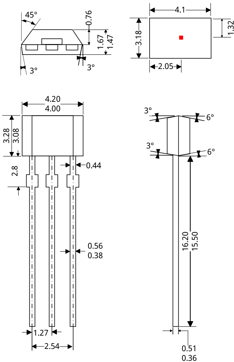
3-脚 A2 封装
