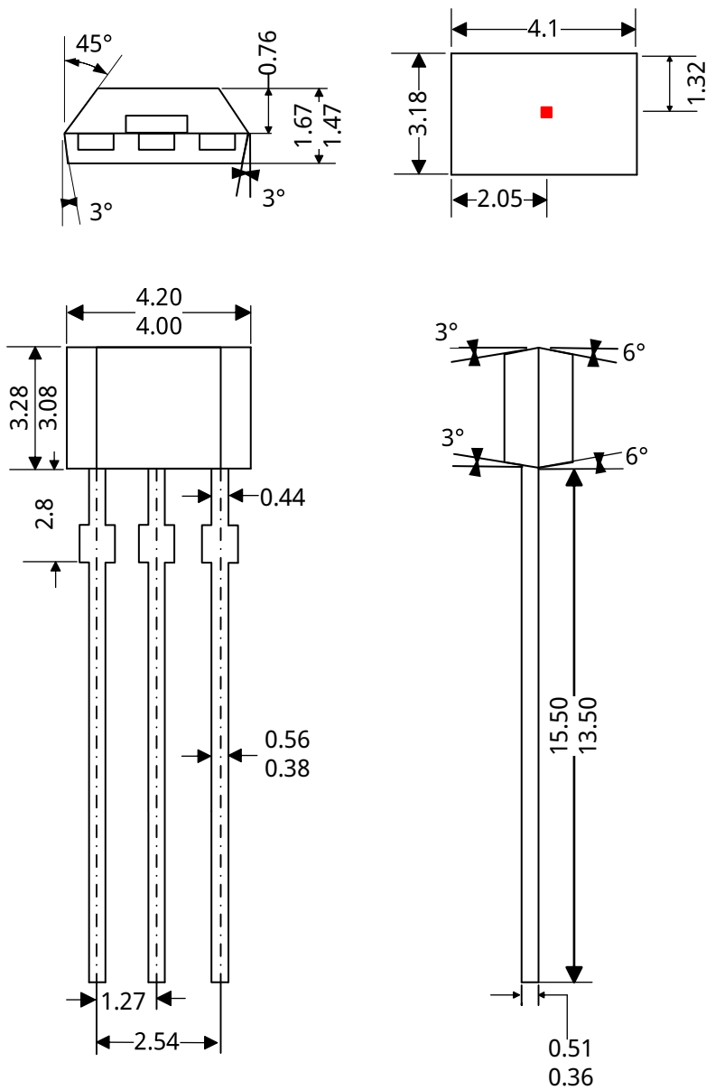
3-脚 A1 封装
