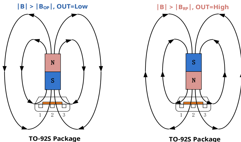
图 4 磁场方向定义图
