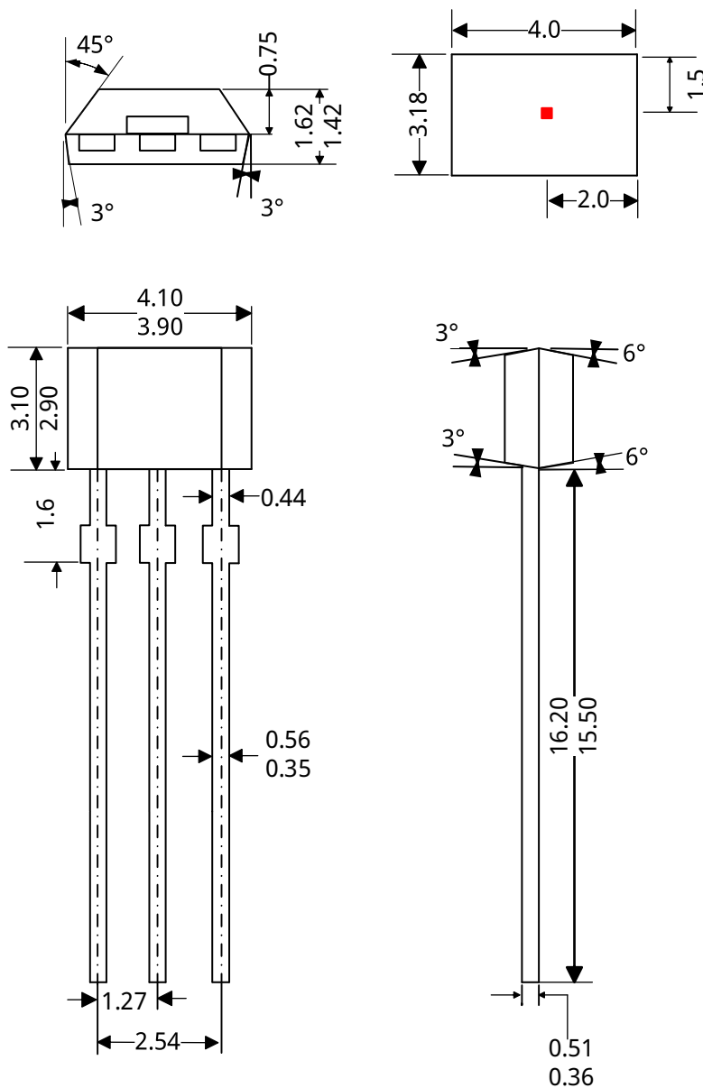
3-脚 B2 封装
