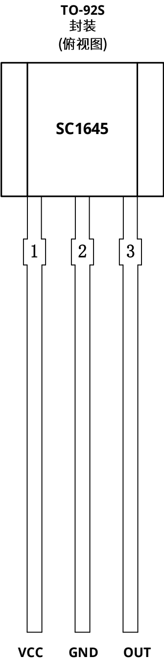
图 2 引脚描述
