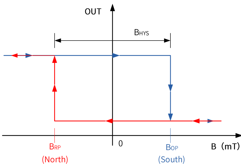
图 5 传输函数图
