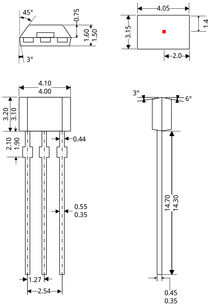
3-脚 S1 封装
