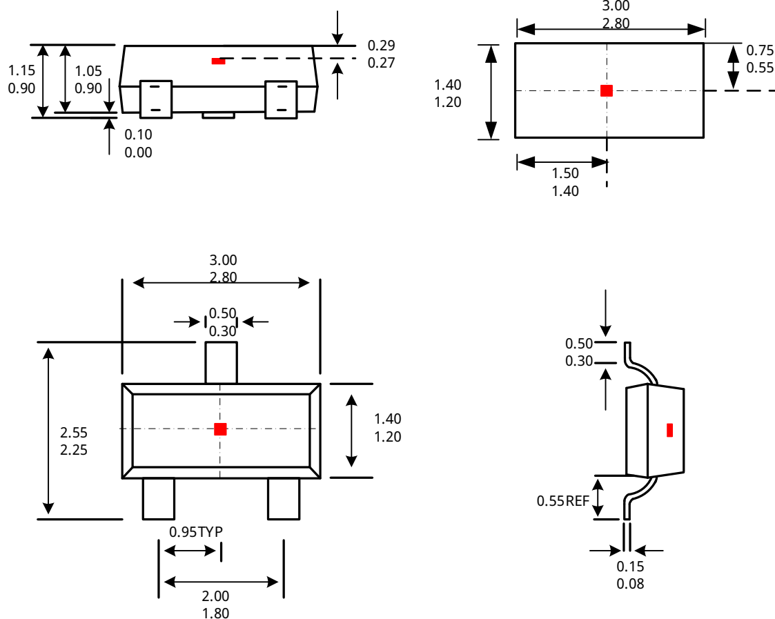
3-Terminal SE Package
