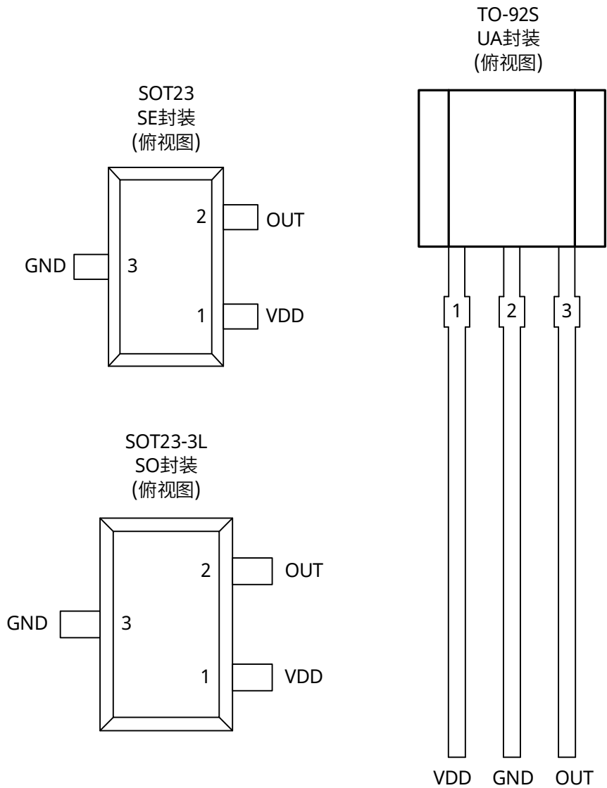
图 2 引脚定义图
