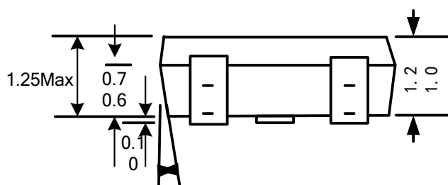
3-脚 SOT23-3L 封装
