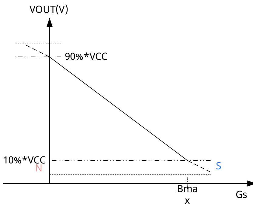
图 8. 输出函数
