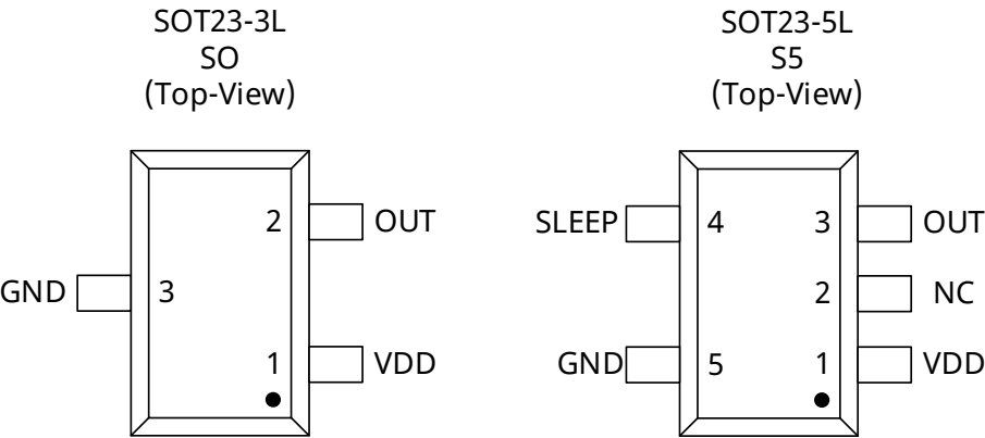
图 2. SOT23-3L 封装俯视图(左) & SOT23-5 封装俯视图(右)
