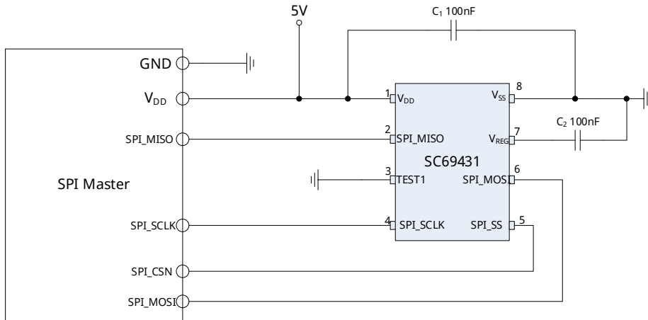
图 32 SPI SOP-8 封装应用参考电路图
