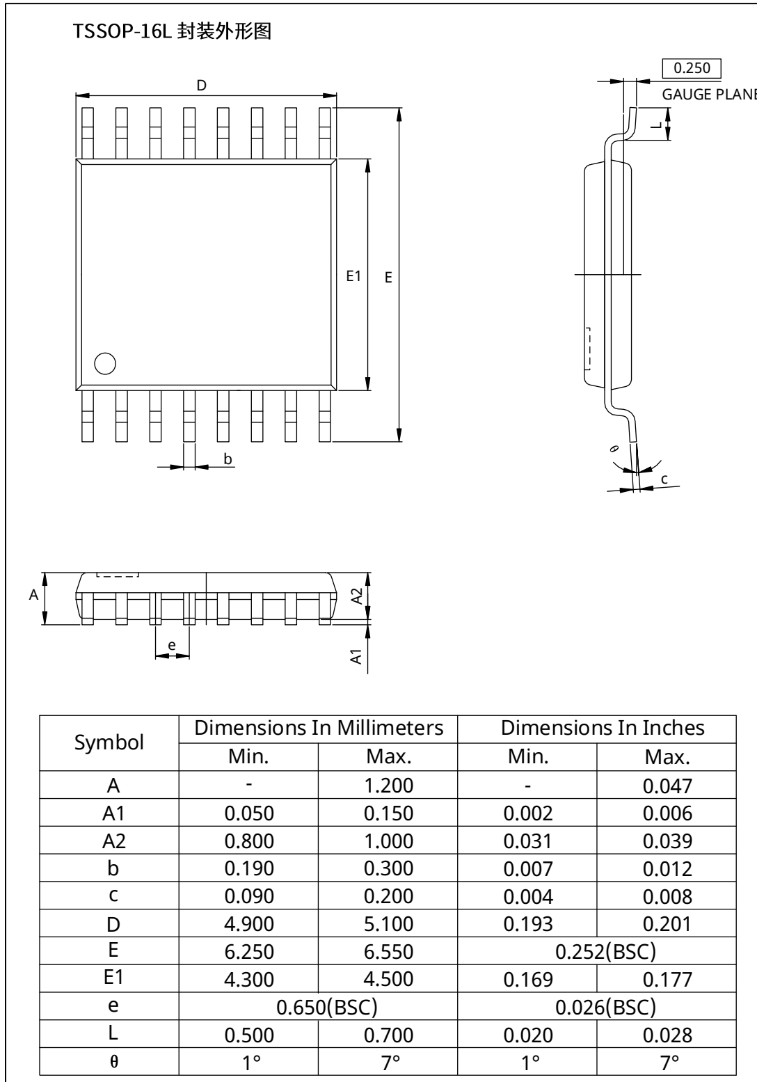
图 36 TSSOP-16 封装尺寸
