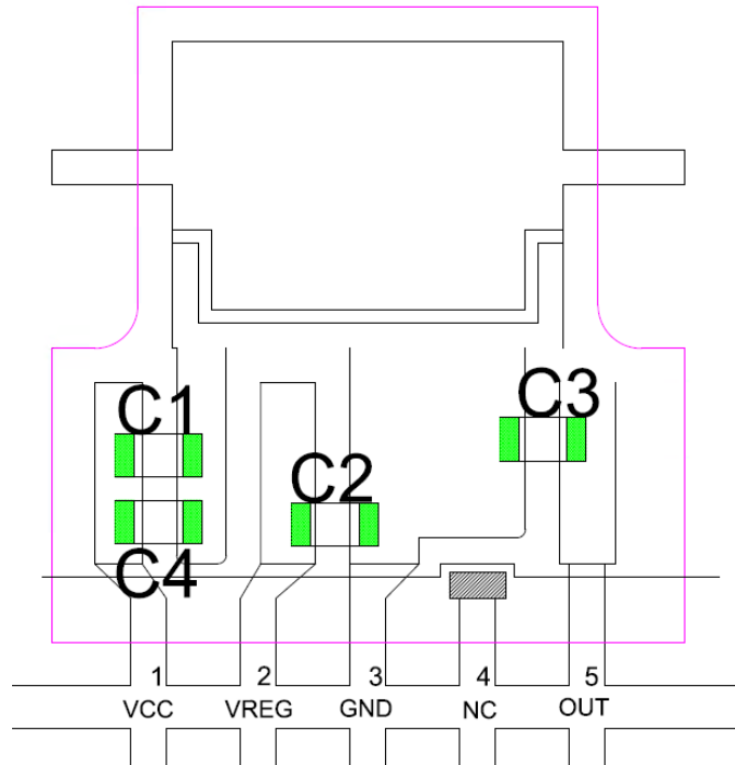
图 34 SIP-3 单芯片封装应用参考电路图
