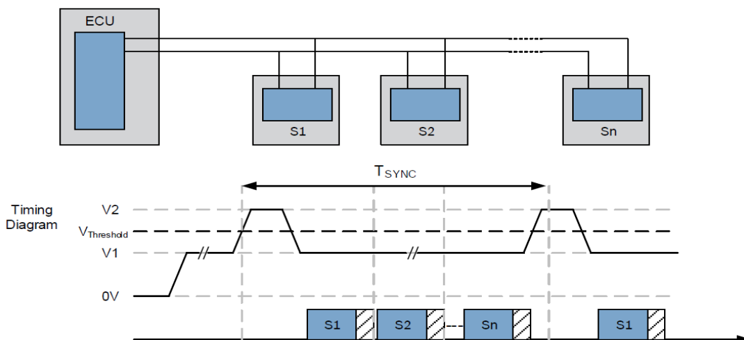
图 21 PSI5 同步并行模式
