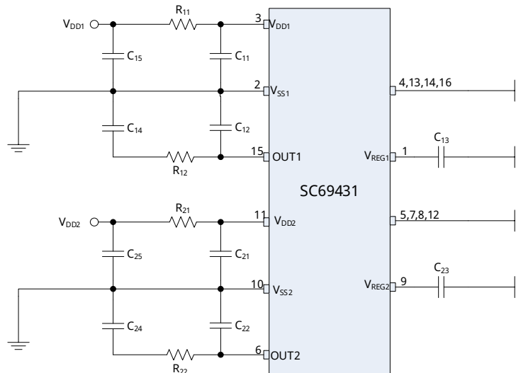
图 29 模拟/PWM TSSOP-16 封装应用参考电路图
