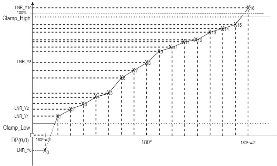
图 26 16 段校准曲线图
