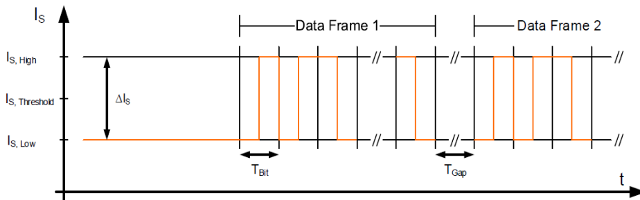
图 19 PSI5 数据电流调制
