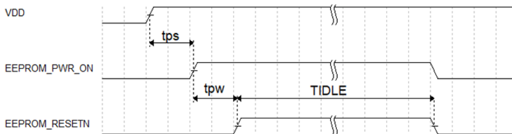
图8 EEPROM时序
