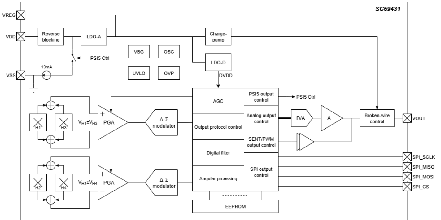
图 10 功能框图
