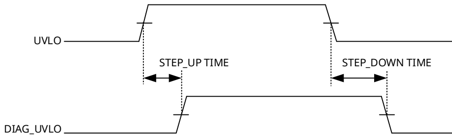
图 22 诊断去抖动时序
