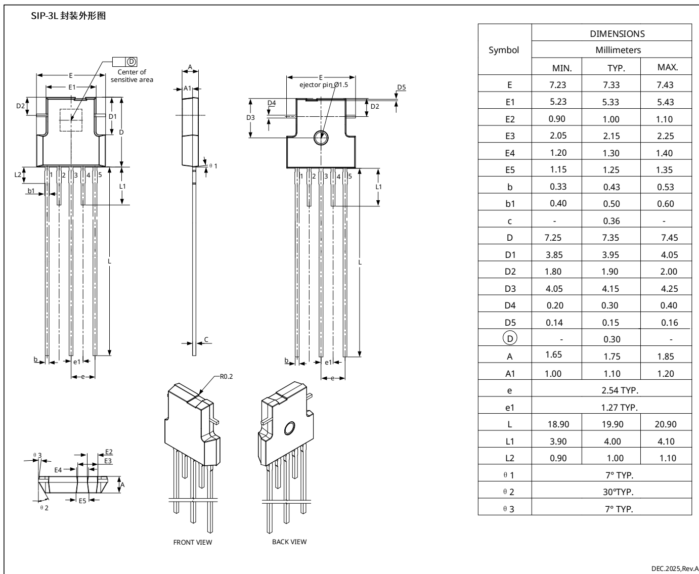
图 37 SIP-3 封装尺寸
