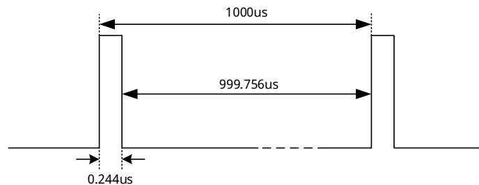
图 12 PWM_POL=1 时PWM输出波形
