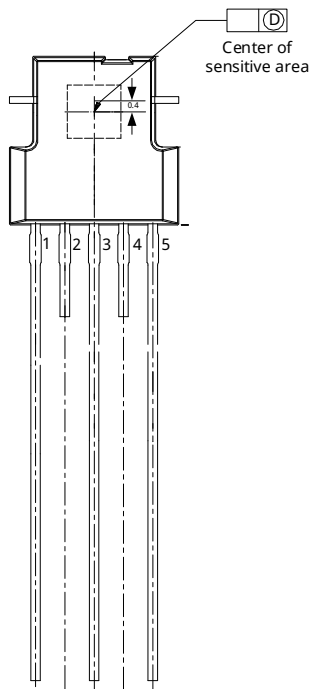
图 5 SIP-3 引脚描述
