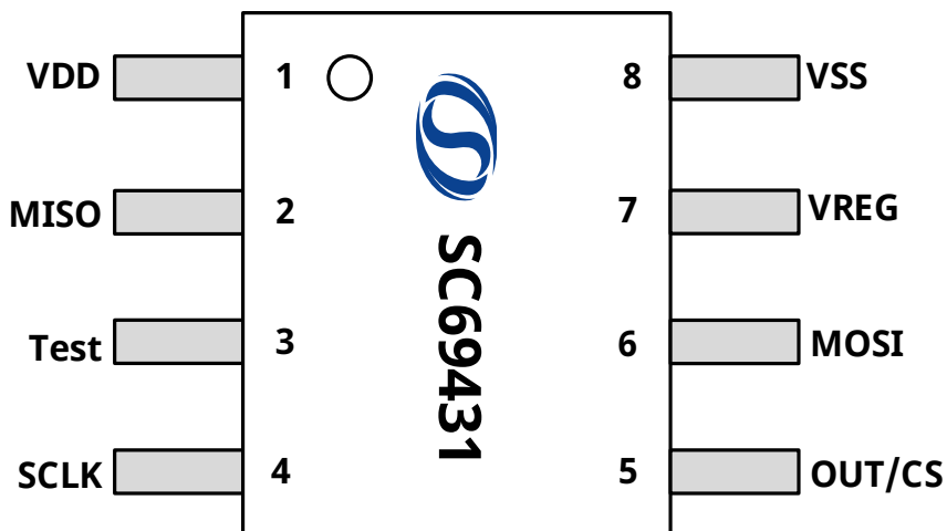
图 3 SOP-8 引脚描述
