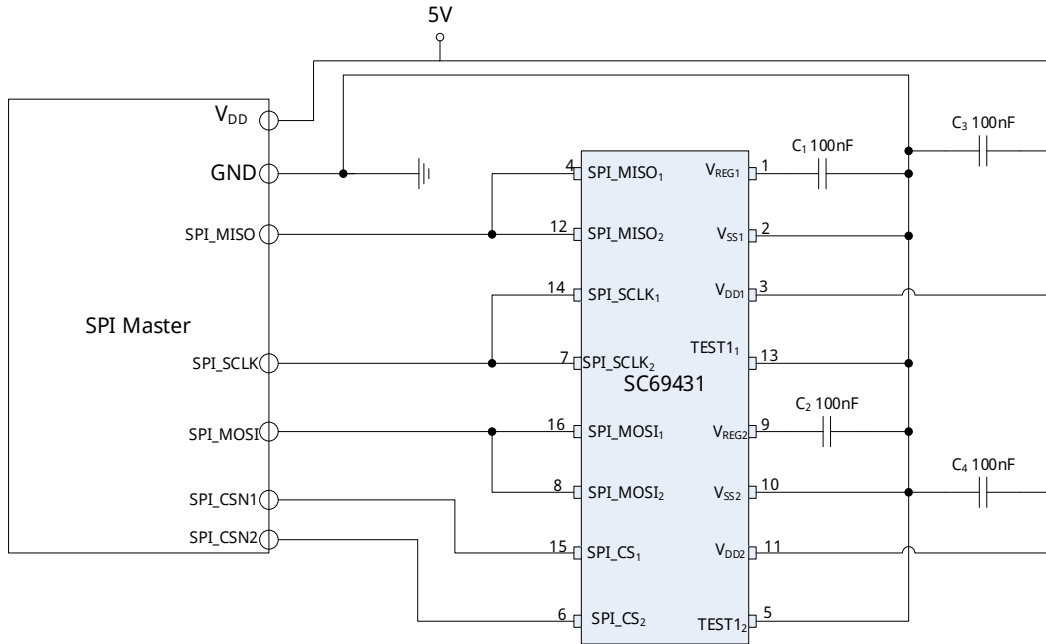
图 33 SPI TSSOP-16 封装应用参考电路图
