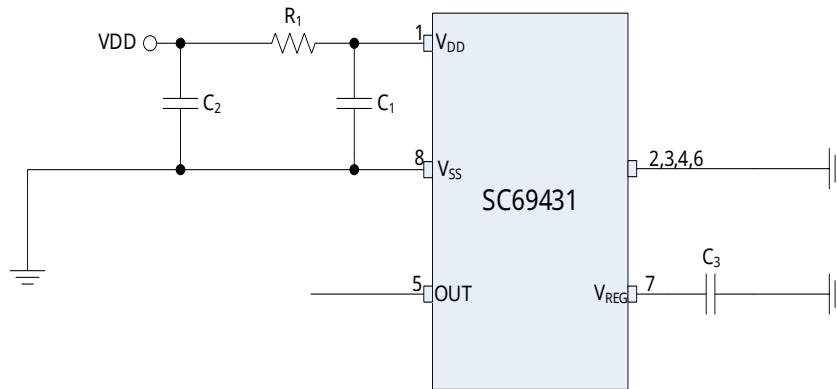
图 30 PSI5输出 SPO-8 封装应用参考电路图
