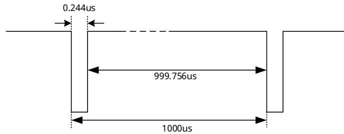
图 11 PWM_POL=0 时PWM输出波形
