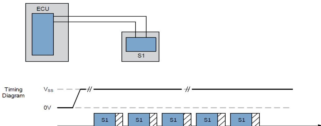
图 20 PSI5 异步模式
