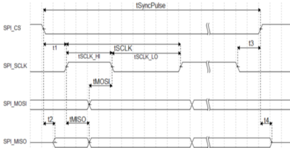
图9 SPI 时序
