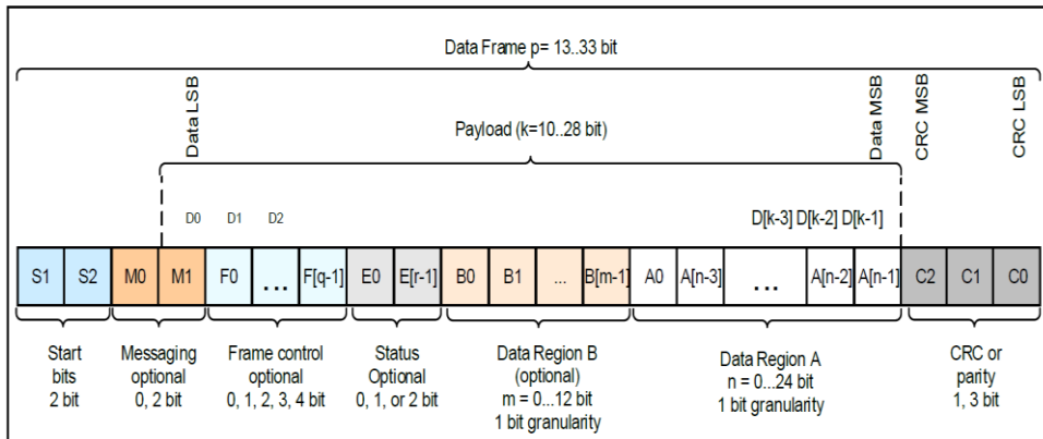
图 18 PSI5 数据帧格式
