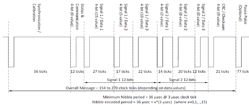
图 13 2通道12位数据SENT信息格式例子
