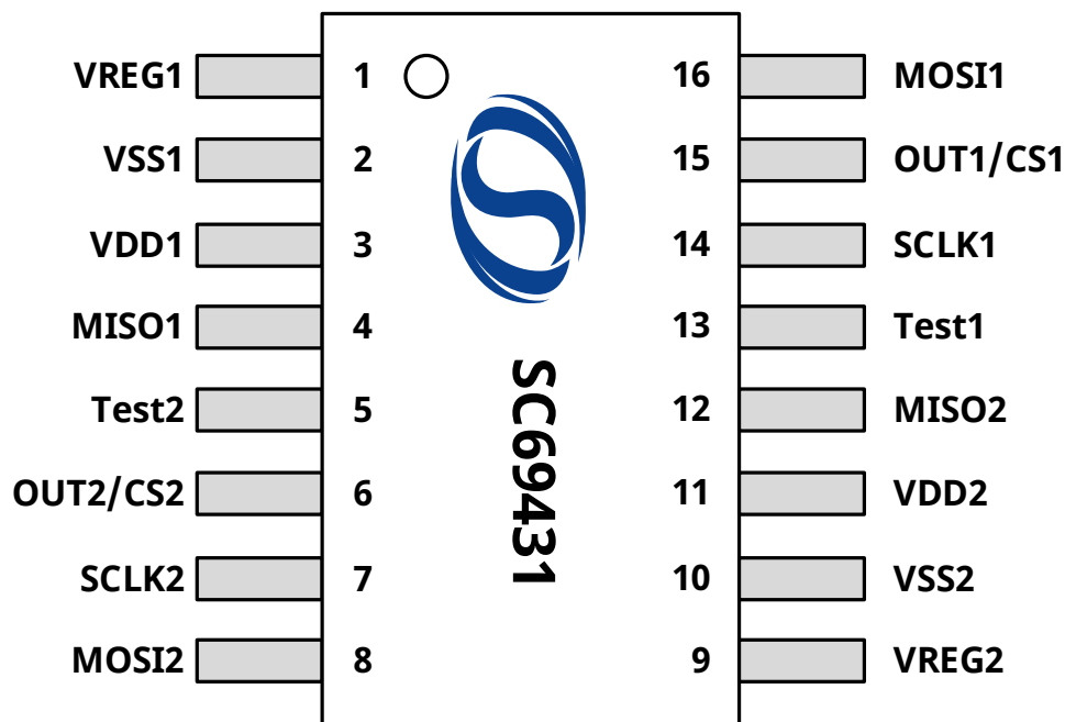
图 4 TSSOP-16 引脚描述
