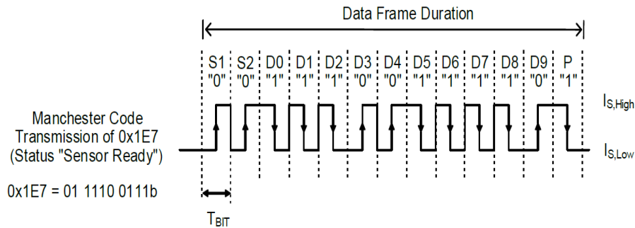
图 17 PSI5 曼彻斯特编码格式
