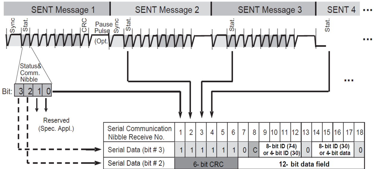
图 16 增强型串行消息数据格式
