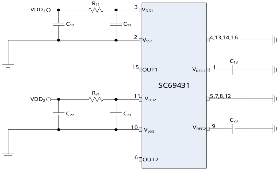
图 31 PSI5 TSSOP-16 输出封装应用参考电路图
