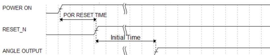
图7 上电复位时序
