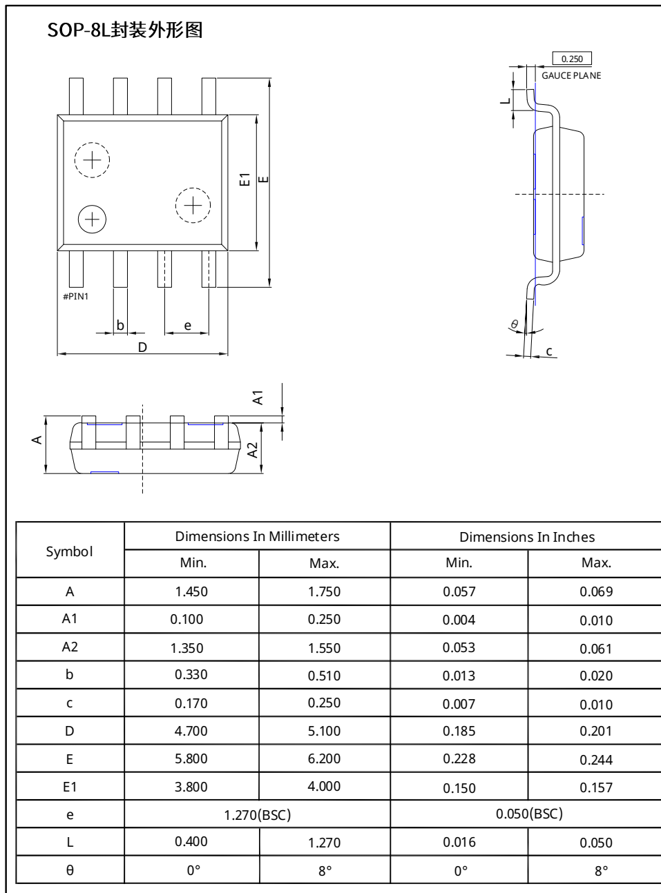
图 35 SOP-8 封装尺寸
