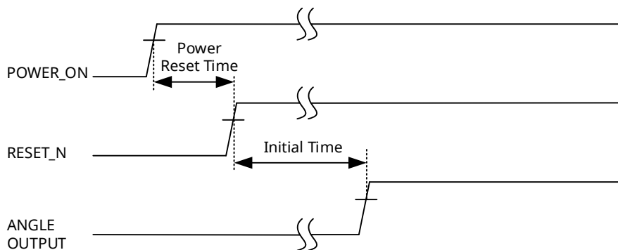
图5: 电复位时序
