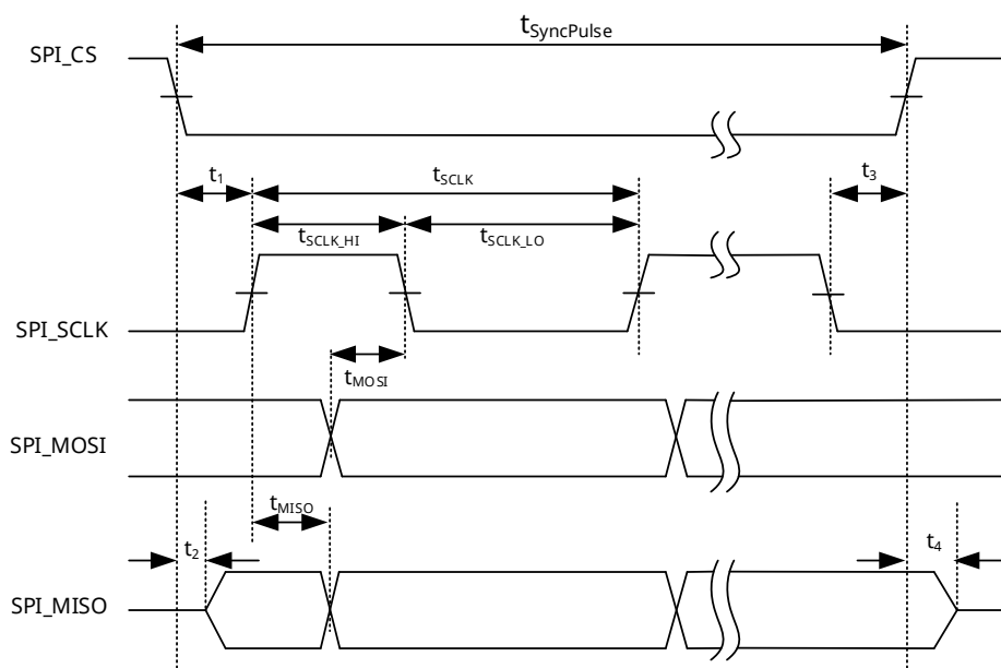
图7: SPI时序
