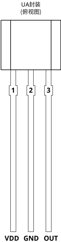
图 2 引脚描述
