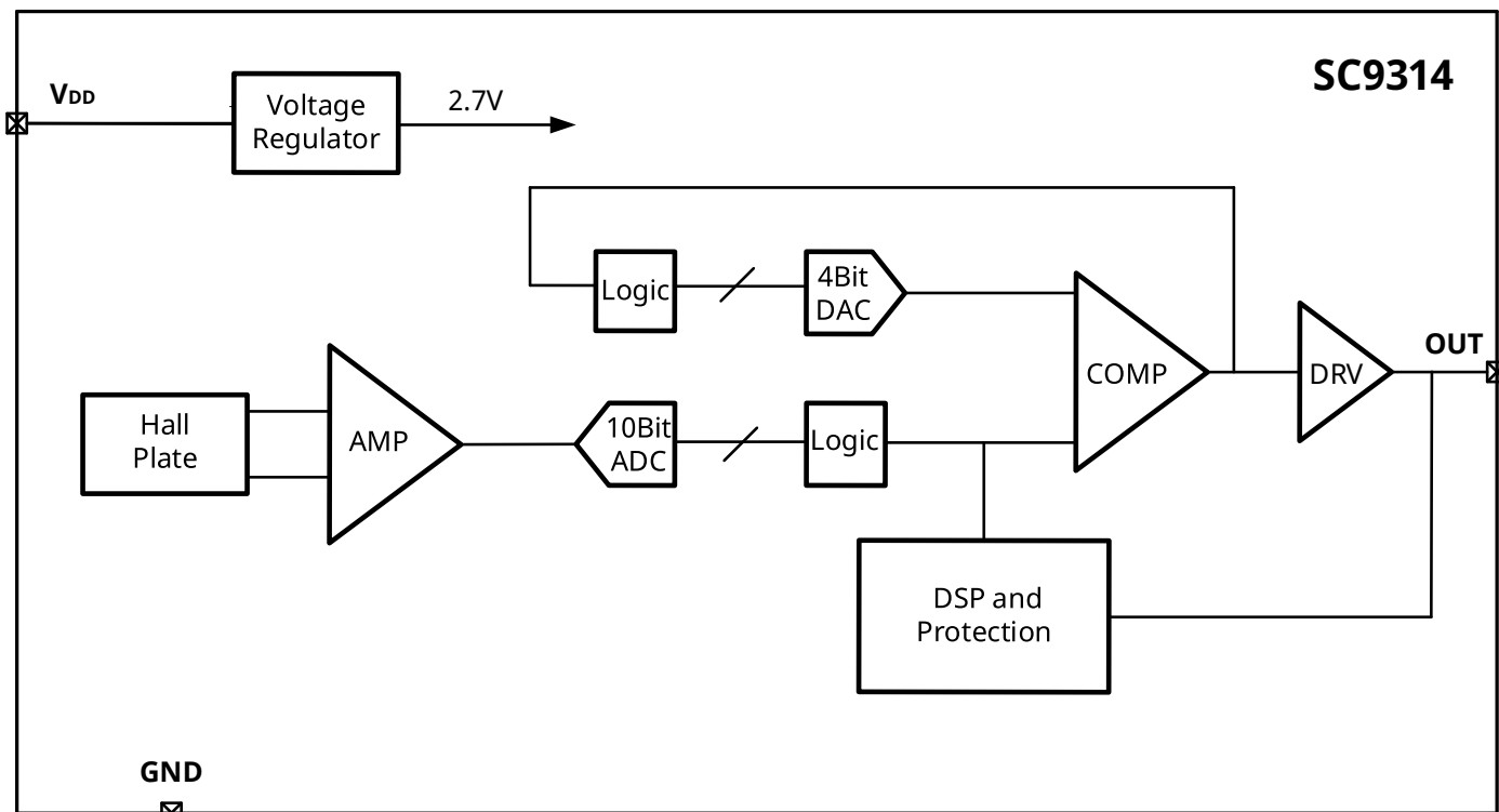
图 3 功能框图
